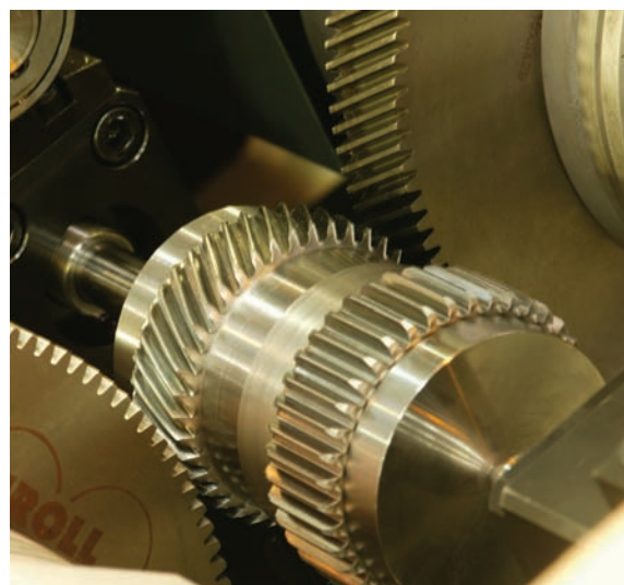
Herstellung von Getriebezahnrädern durch Profilwalzen
