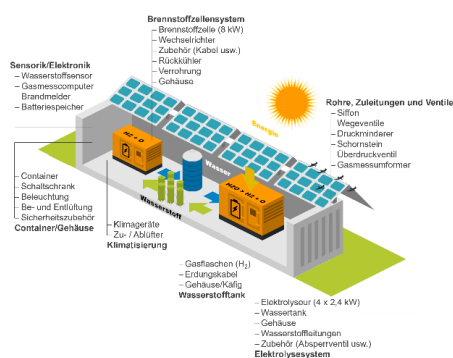
Abb. 2 Struktur und Kernkomponenten eines Microgrids
